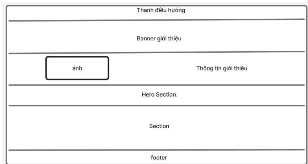
Hình 3.3 Layout giao diện trang giới thiệu
