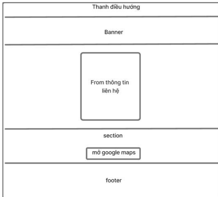
Hình 3.4 Layout giao diện trang liên hệ
