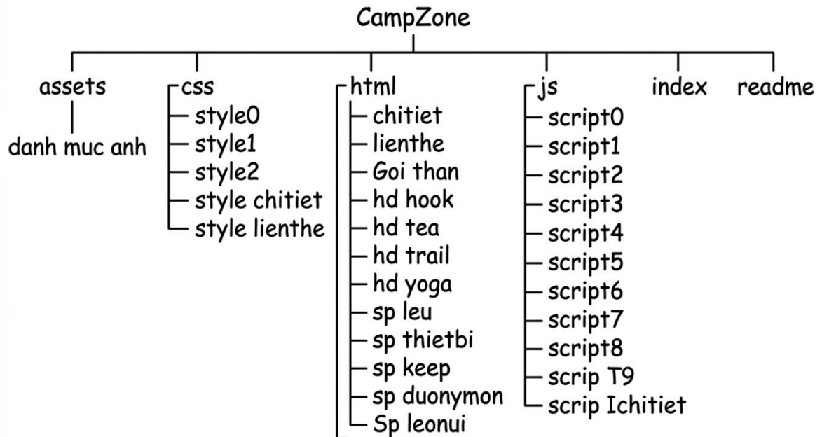
Hình 3.1 Sơ đồ website Campzone
